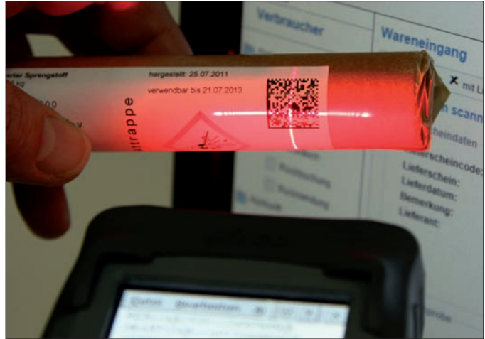
Kennzeichnung und Rückverfolgung: Sprengstoffpakete mit Code; Einscannen einer Sprengpatrone.
